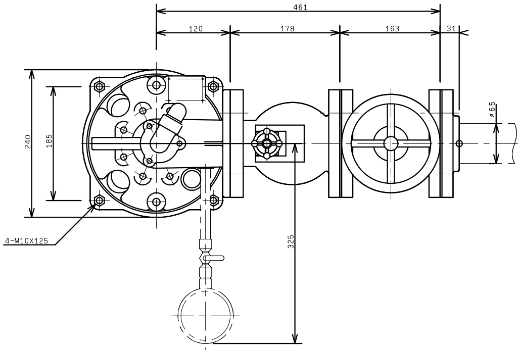
平面図
