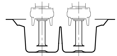
ベルマウス詳細図
