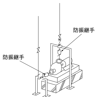
形鋼振れ止め支持の例
