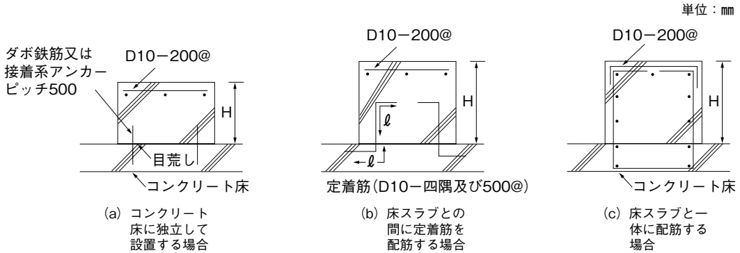
[基礎の高さと配筋要領]
