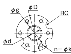
口径50mm
