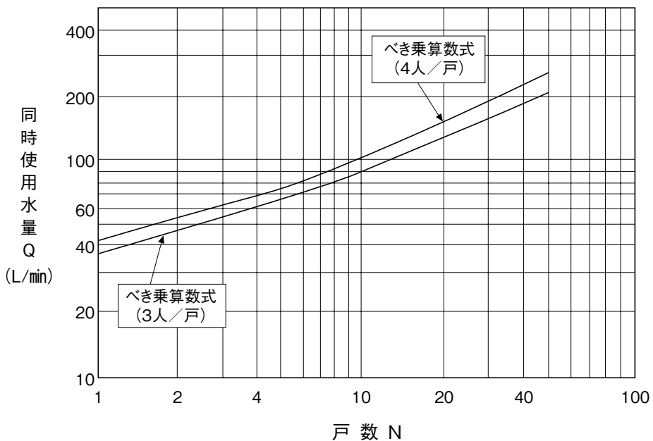
給水戸数と同時使用水量
