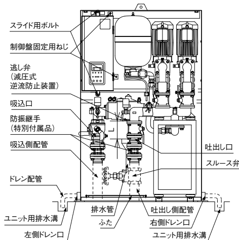
垂直配管の場合
