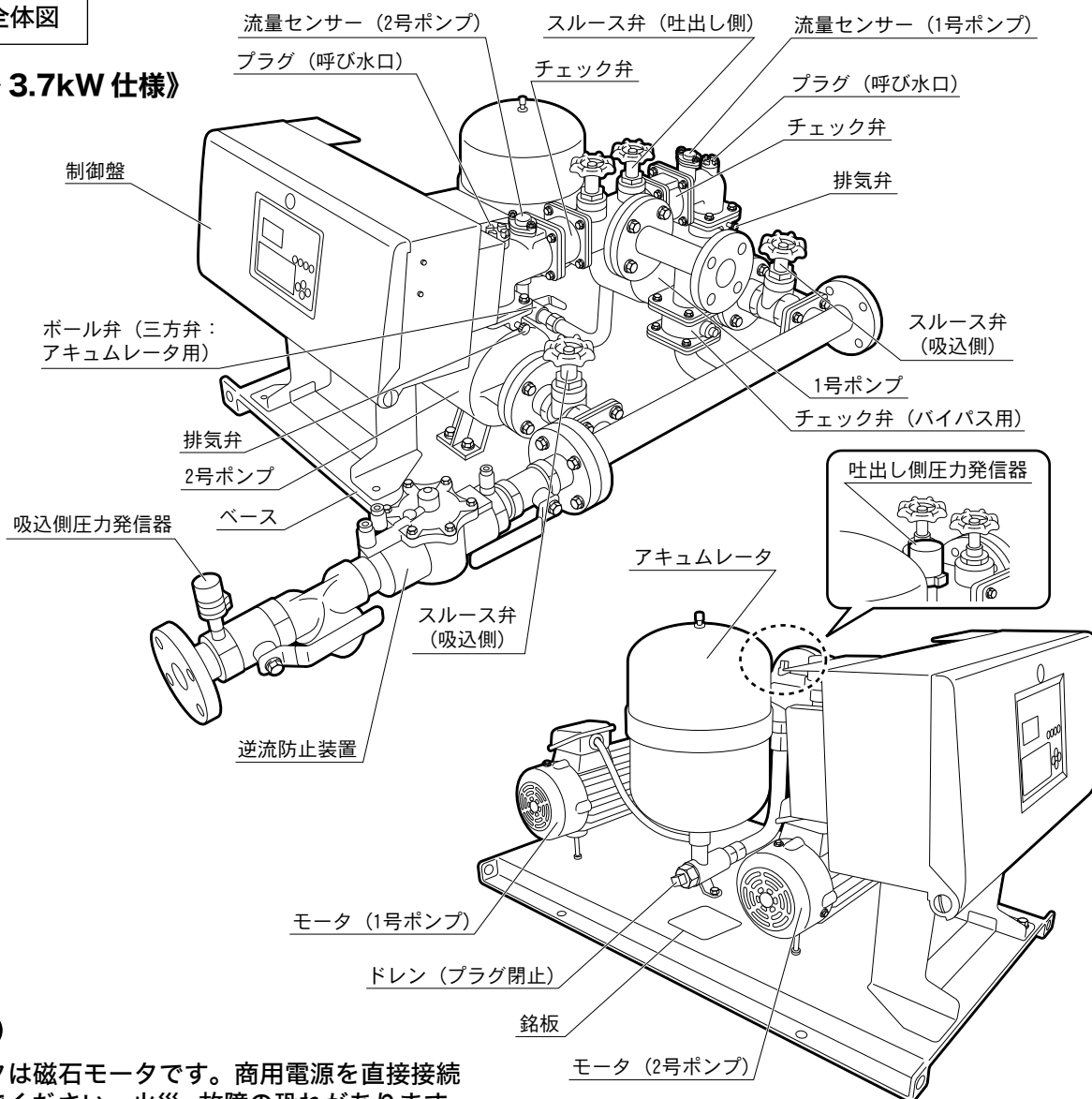
製品全体図
