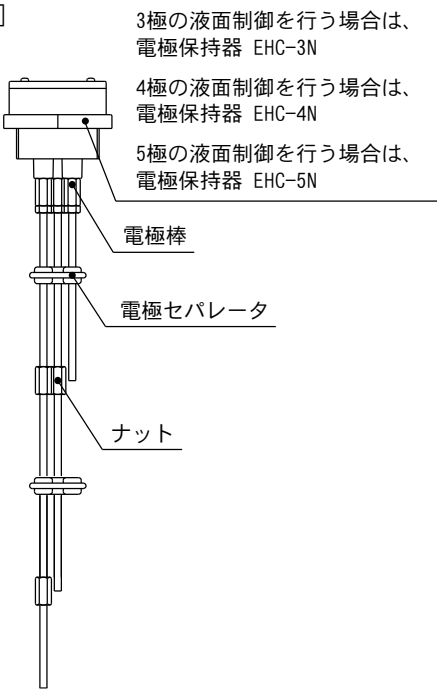
〔電極棒〕
