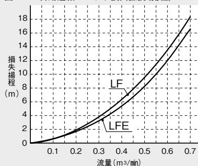
図-1 自動運転ユニット損失抵抗(揚程)
