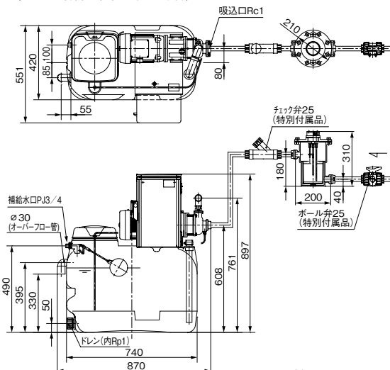
(VC80:制御盤位置変更の場合)
