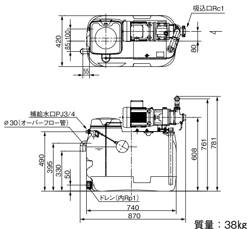
DW2-25CE0.75+受水槽TAB-5の例
