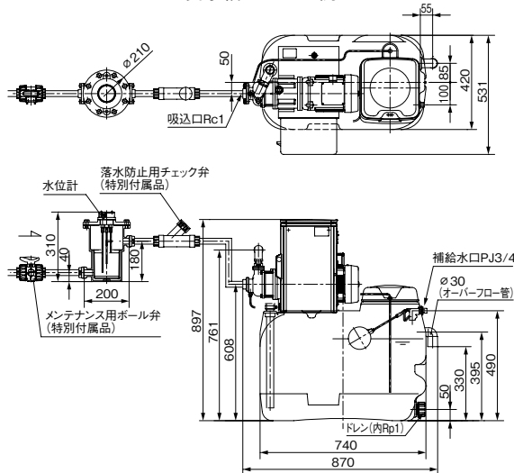
DW2-25SE0.75+受水槽TAB-5の例
