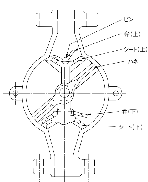
A-A断面
