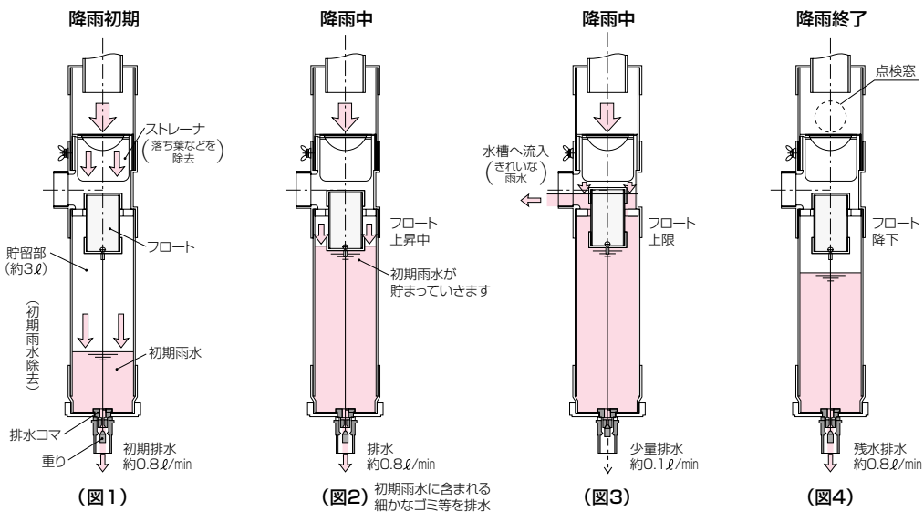
図は、雨の降り始めから、雨が止むまでのセパレータの水位、フロート、重りの動きを示したものです。
