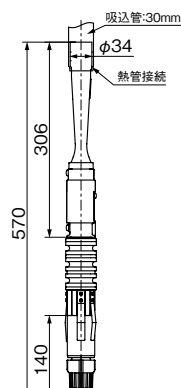
φ50ステンレス製 シングルジェット
