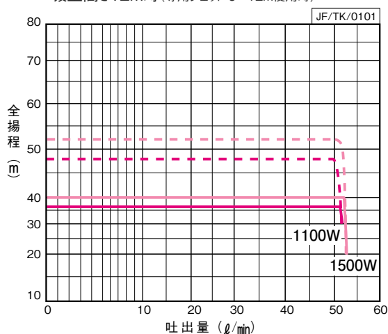
吸上高さ12m時(専用ジェット 6~12m使用時)
