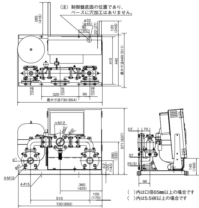
[自動運転ユニット部UF形寸法図]
