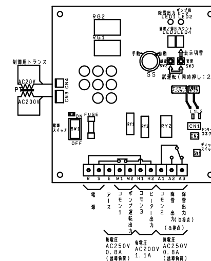
制御盤 結線図
