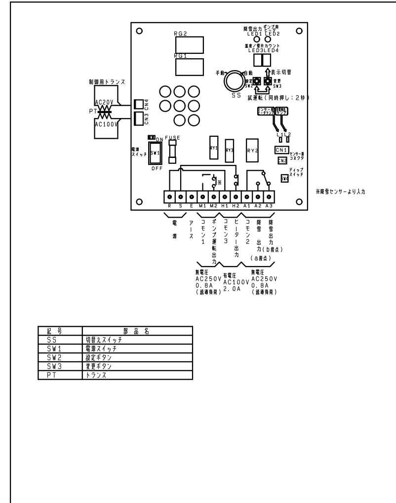
制御盤 結線図
