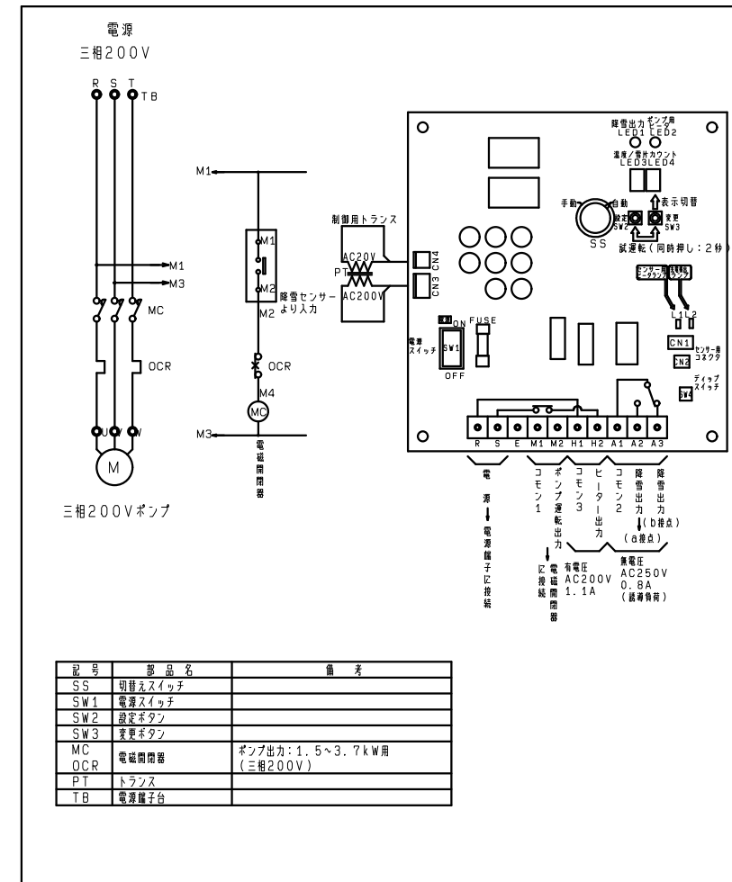
制御盤 結線図
