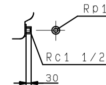
排水口詳細
