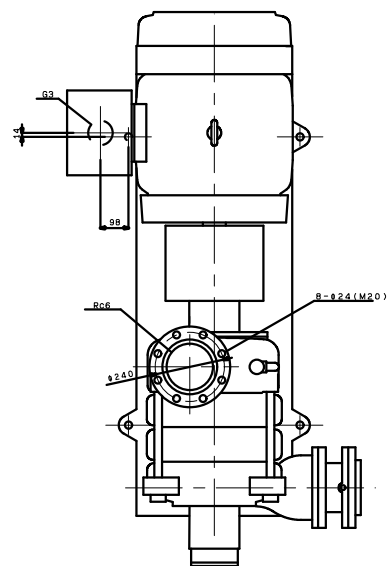
TVS1506X3ME75 (VC30)
