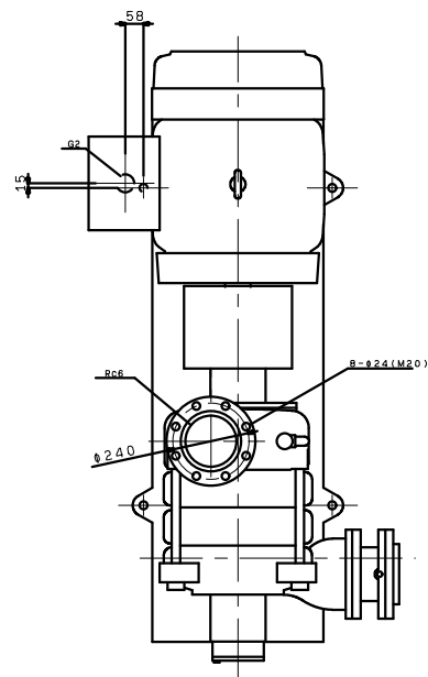
TVS1505X3ME55 (VC30)
