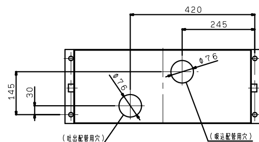
矢視Z (本体下部詳細)
