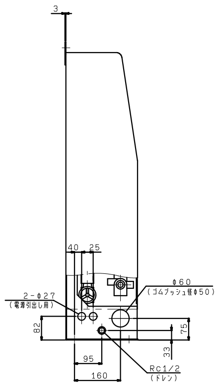
矢視Z (本体下部詳細)
