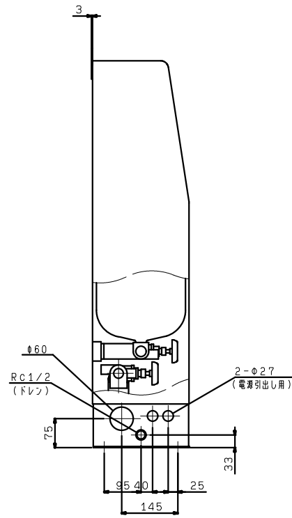
矢視A (本体下部詳細)
