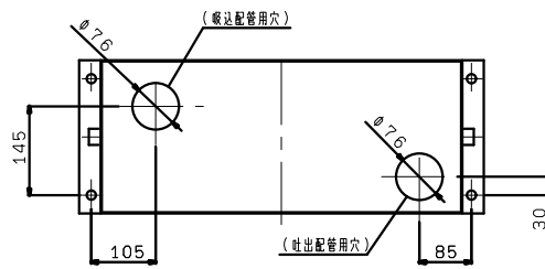
矢視A (本体下部詳細)
