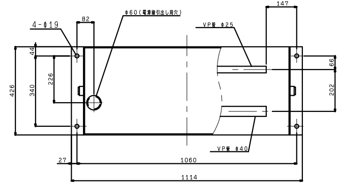
A-A (下部詳細)
