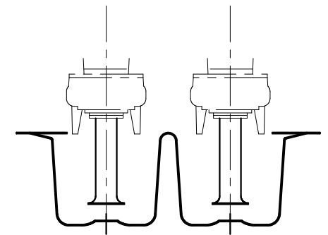
ベルマウス詳細図
